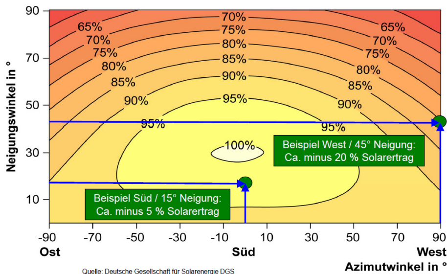
Solarertrag in % (Solarthermie)
