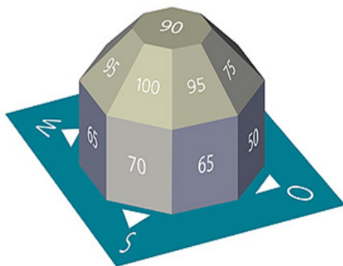
Solarertrag in % (Solarthermie)
